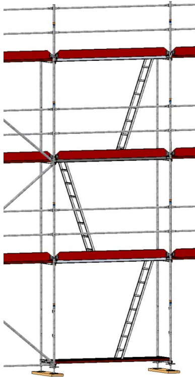
Bild 49: Innenliegender Leitergang
