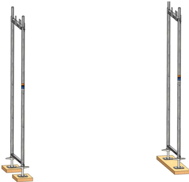
Bild 6: Aufbau des ersten Gerüstfeldes: Vertikalrahmen
